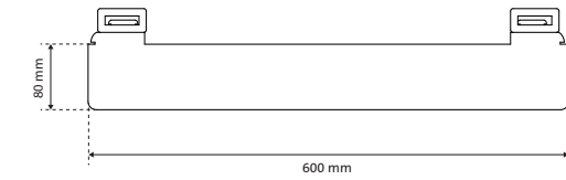
Zijaanzicht V2
