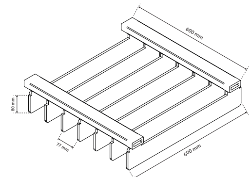
Bovenaanzicht V2
