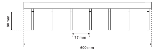
Vooraanzicht V2
