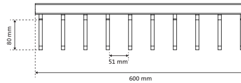
Vooraanzicht V1
