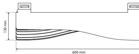
Zijaanzicht V1
