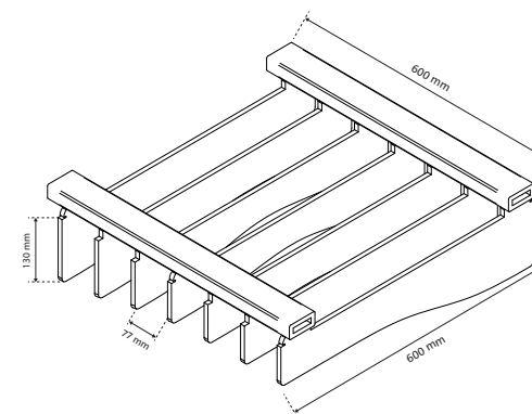
Bovenaanzicht V2
