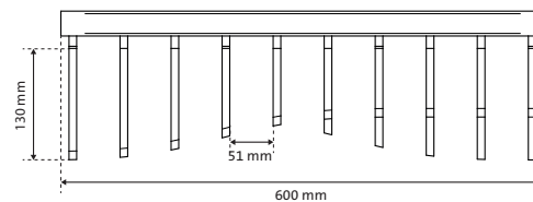
Vooraanzicht V1
