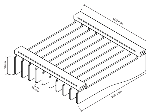
Bovenaanzicht V1
