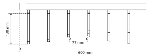
Vooraanzicht V2
