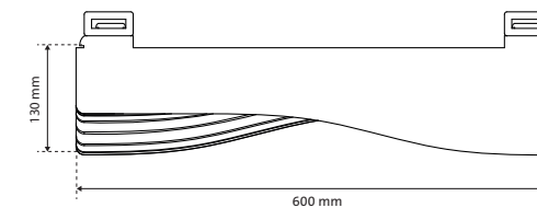
Zijaanzicht V2
